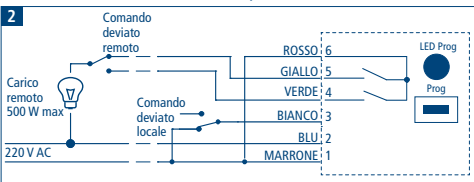
Nuovo collegamento con RX Domotico alimentazione 220 V AC (2x500W) modalità 1D
