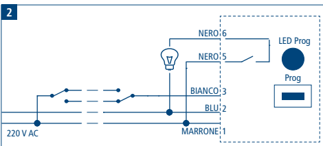
Nuovo collegamento con RX Domotic alimentazione 220 V AC 1 uscita
